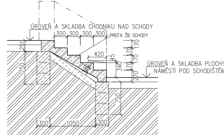
ŘEZ D1-D1'
