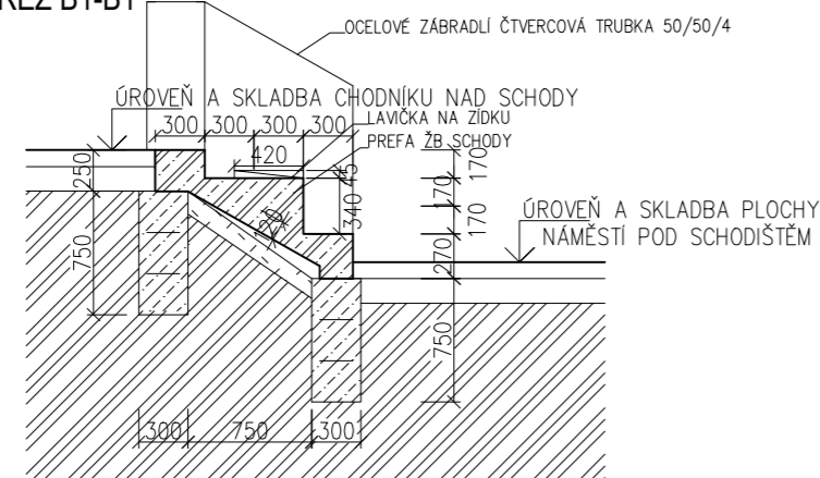
ŘEZ B1-B1'
