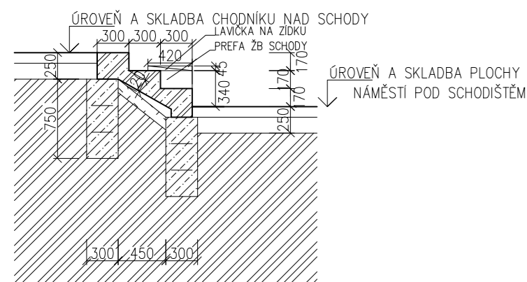
ŘEZ A2-A2'
