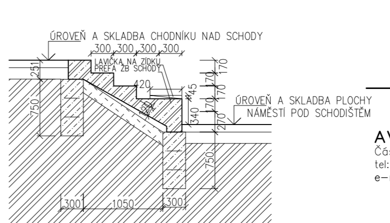
ŘEZ D2-D2'
