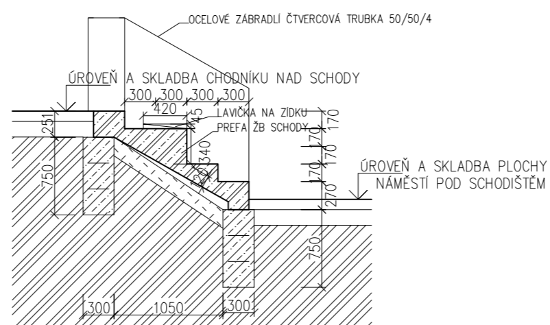
ŘEZ C1-C1'
